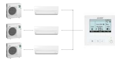
Fonction secours
